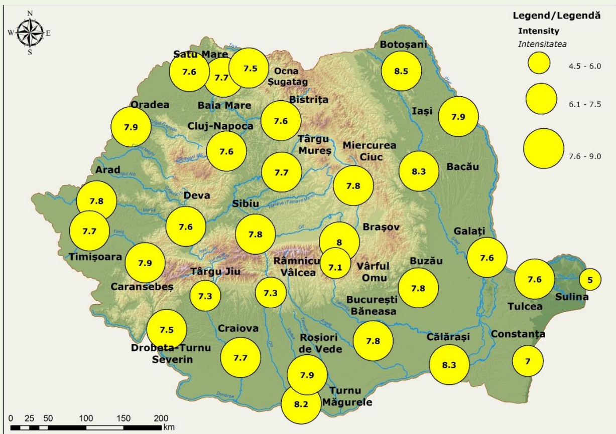
Fig. 1.50. Spatial distribution of mean annual intensity of moderate heat waves/warm spells Distribuția spațială a intensității medii anuale a valurilor de căldură/periodelor calde moderate
