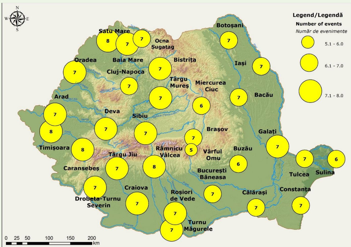
Fig. 1.52. Spatial distribution of mean annual number of moderate heat waves/warm spells Distribuția spațială a numărului medii anuale al valurilor de căldură/periodelor calde moderate
