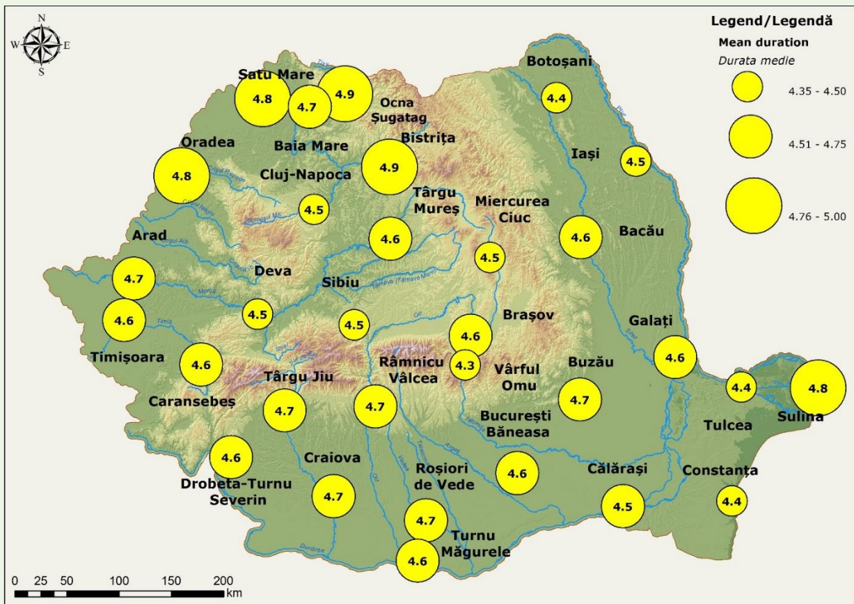
Fig. 1.51. Spatial distribution of mean annual duration of moderate heat waves/warm spells Distribuția spațială a duratei medii anuale a valurilor de căldură/periodelor calde moderate
