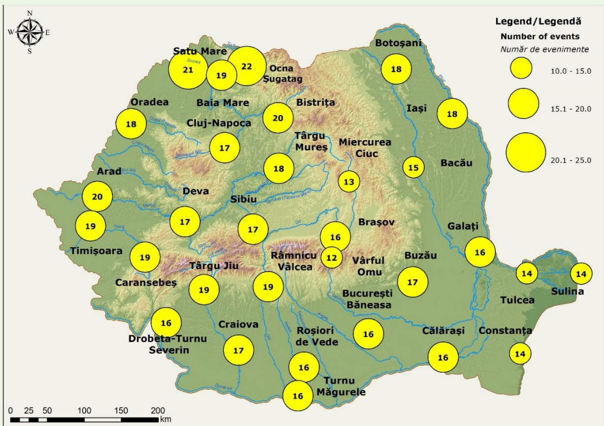
Fig. 1.48. Spatial distribution of maximum annual number of moderate heat waves/warm spells Distribuția spațială a numărului maxim anual al valurilor de căldură/perioadelor calde moderate
