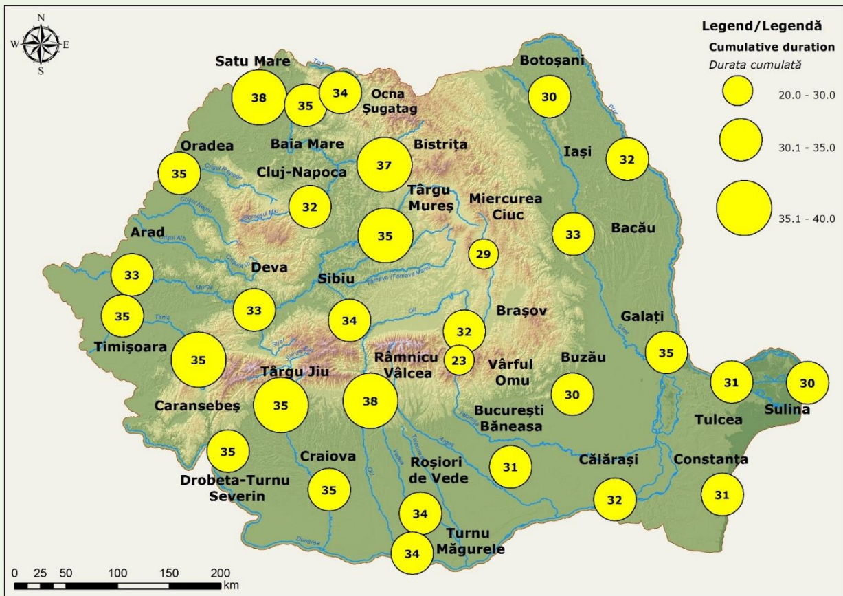
Fig. 1.49. Spatial distribution of mean annual cumulative duration of moderate heat waves/warm spells Distribuția spațială a duratei cumulate medii anuale a valurilor de căldură/periodelor calde moderate
