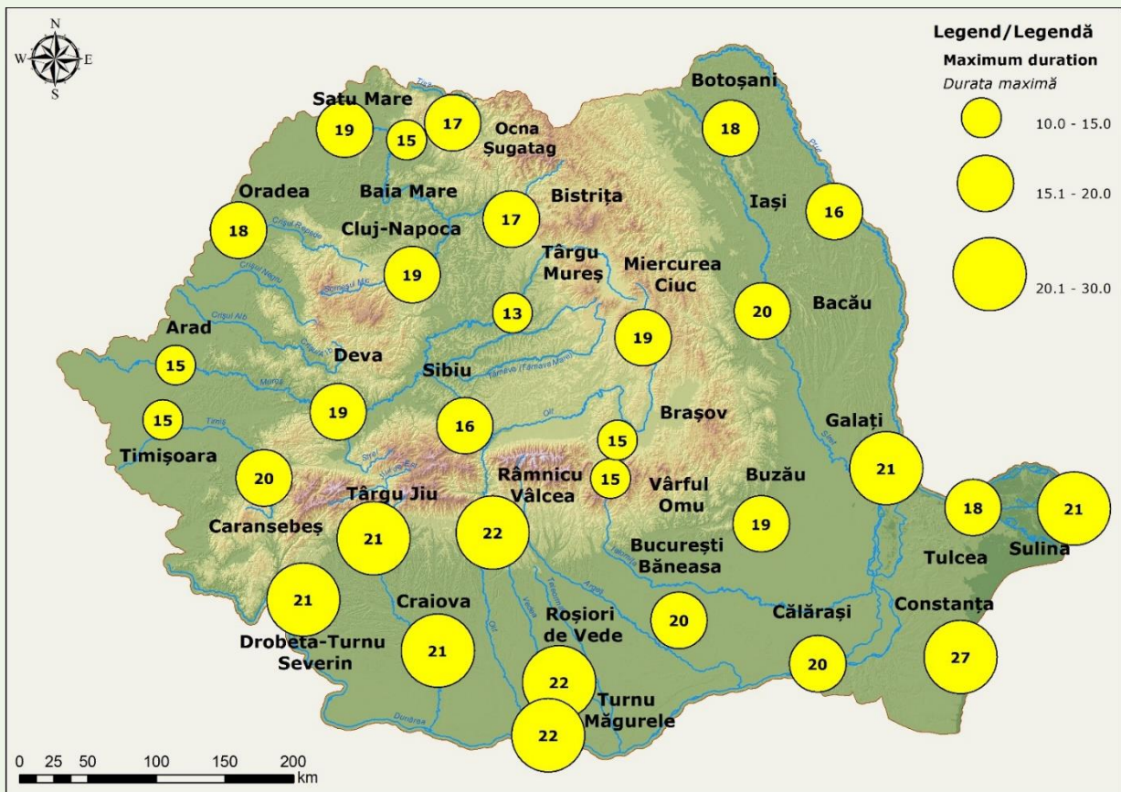
Fig. 1.47. Spatial distribution of maximum annual duration of moderate heat waves/warm spells Distribuția spațială a duratei maxime anuale a valurilor de căldură/perioadelor calde moderate
