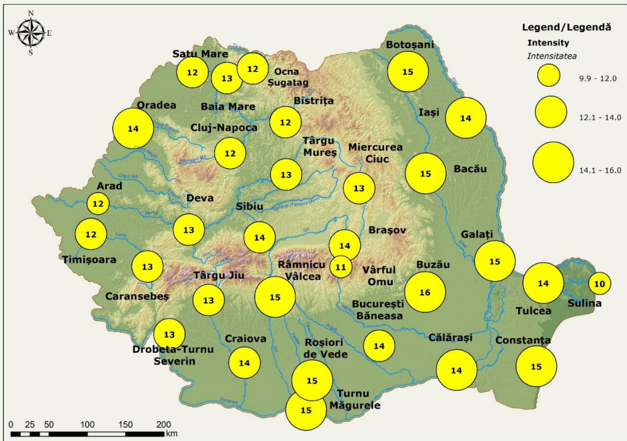
Fig. 1.46. Spatial distribution of maximum annual intensity of moderate heat waves/warm spells Distribuția spațială a intensității maxime anuale a valurilor de căldură/periodelor calde moderate
