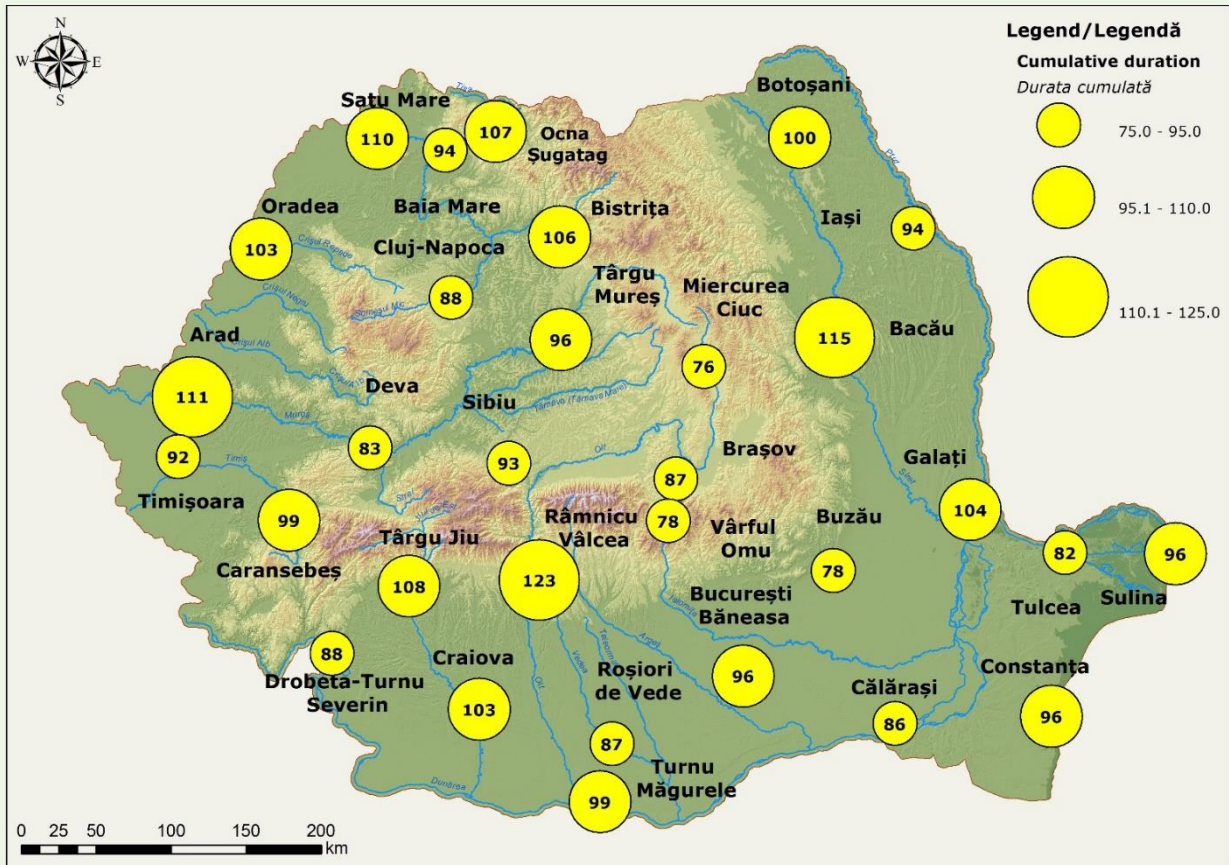
Fig. 1.45. Spatial distribution of maximum annual cumulative duration of moderate heat waves/warm spells Distribuția spațială a duratei cumulate maxime anuale a valurilor de căldură/periodelor calde moderate
