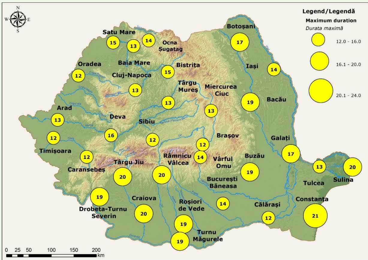
Fig. 1.87. Spatial distribution of maximum annual duration of severe heat waves/warm spells Distribuția spațială a duratei maxime anuale a valurilor de căldură/perioadelor calde severe
