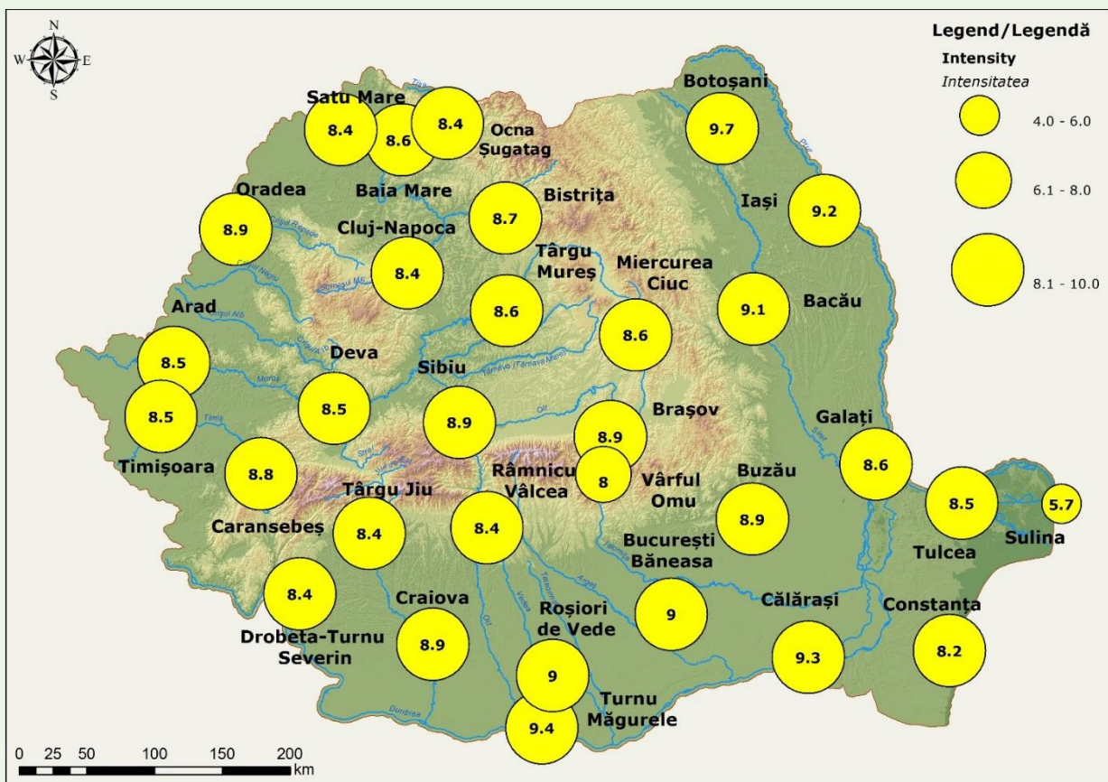
Fig. 1.90. Spatial distribution of mean annual intensity of severe heat waves/warm spells Distribuția spațială a intensității medii anuale a valurilor de căldură/periodelor calde severe
