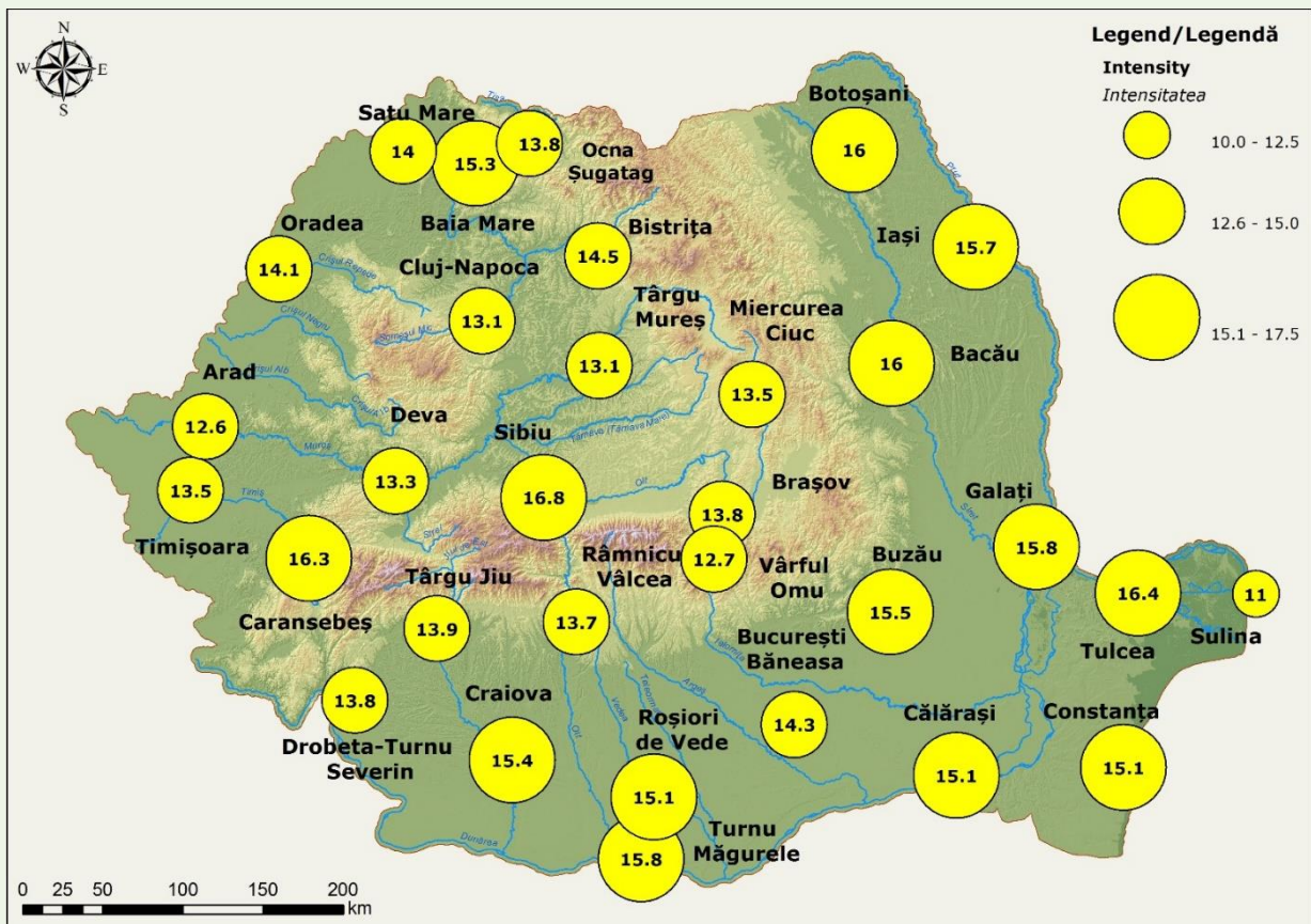
Fig. 1.86. Spatial distribution of maximum annual intensity of severe heat waves/warm spells Distribuția spațială a intensității maxime anuale a valurilor de căldură/perioadelor calde severe
