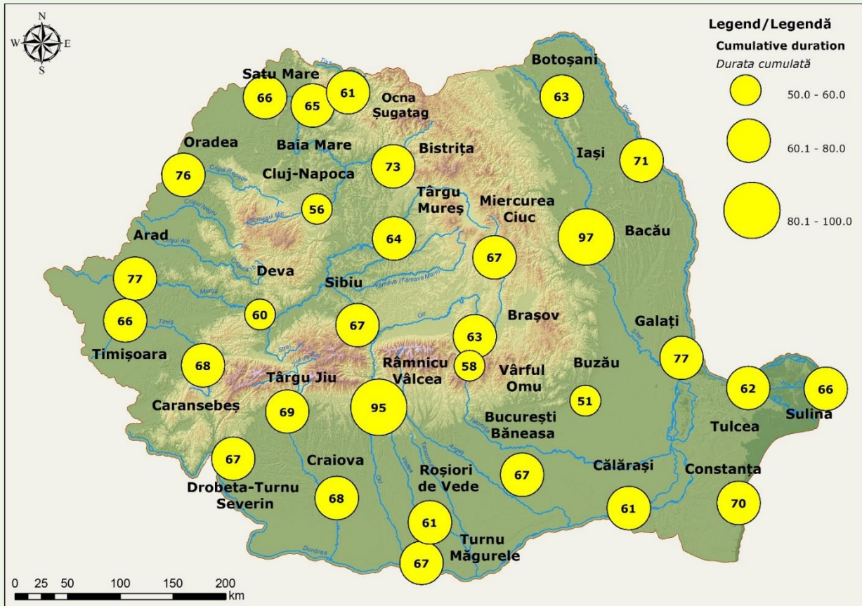
Fig. 1.85. Spatial distribution of maximum annual cumulative duration of severe heat waves/warm spells Distribuția spațială a duratei cumulate maxime anuale a valurilor de căldură/perioadelor calde severe
