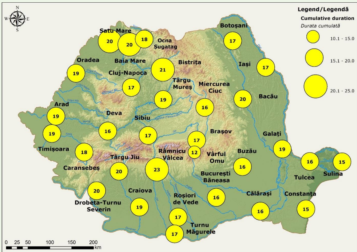
Fig. 1.89. Spatial distribution of mean annual cumulative duration of severe heat waves/warm spells Distribuția spațială a duratei cumulate medii anuale a valurilor de căldură/periodelor calde severe
