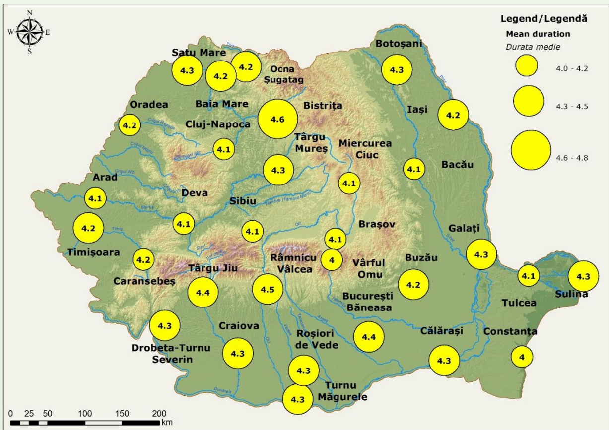
Fig. 1.91. Spatial distribution of mean annual duration of severe heat waves/warm spells Distribuția spațială a duratei medii anuale a valurilor de căldură/periodelor calde severe
