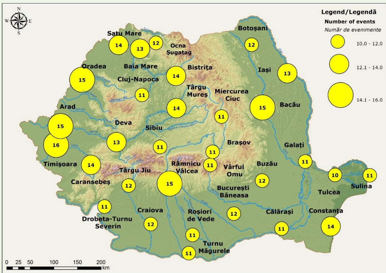
Fig. 1.88. Spatial distribution of maximum annual number of severe heat waves/warm spells Distribuția spațială a numărului maxim anual al valurilor de căldură/perioadelor calde severe
