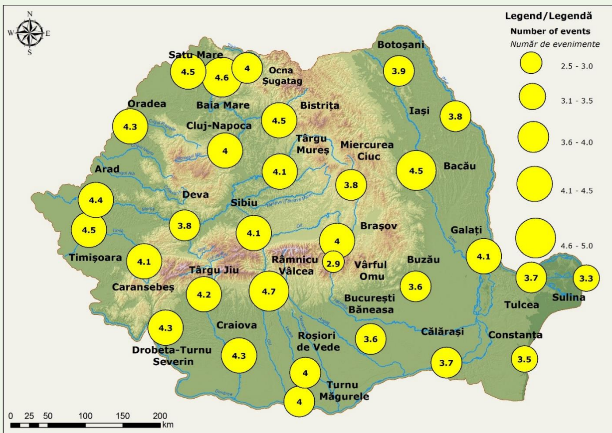
Fig. 1.92. Spatial distribution of mean annual number of severe heat waves/warm spells Distribuția spațială a numărului mediu anual al valurilor de căldură/periodelor calde severe
