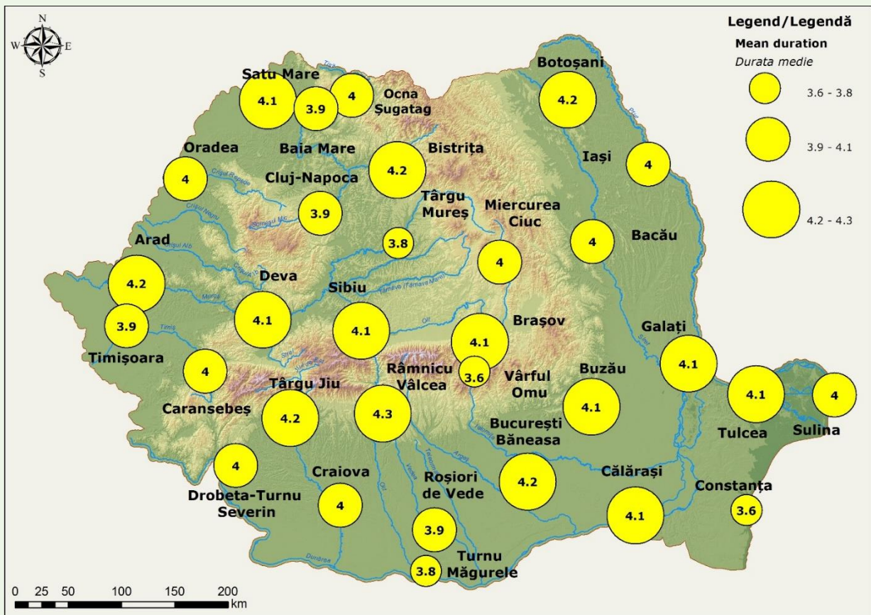
Fig. 1.131. Spatial distribution of mean annual duration of extremely severe heat waves/warm spells Distribuția spațială a duratei medii anuale a valurilor de căldură/perioadelor calde extrem de severe
