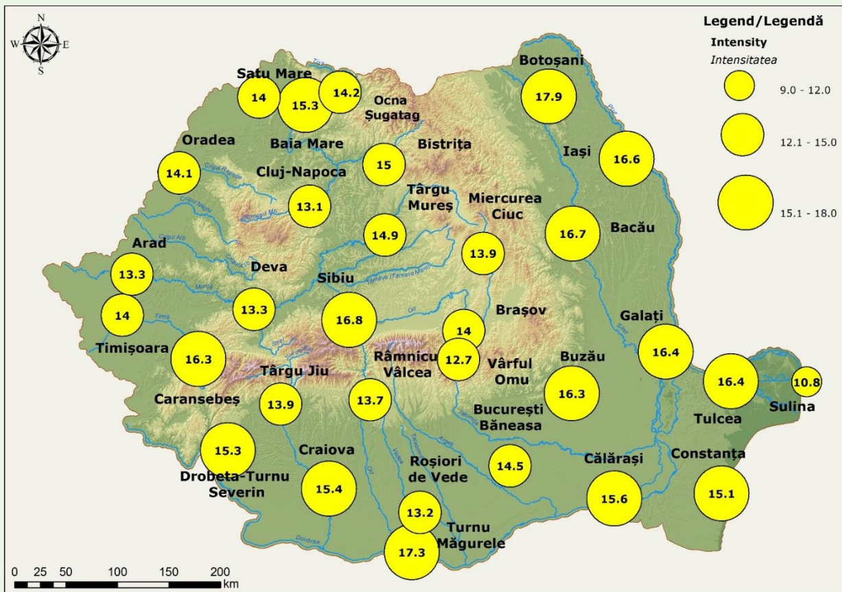
Fig. 1.126. Spatial distribution of maximum annual intensity of extremely severe heat waves/warm spells Distribuția spațială a intensității maxime anuale a valurilor de căldură/periodelor calde extrem de severe
