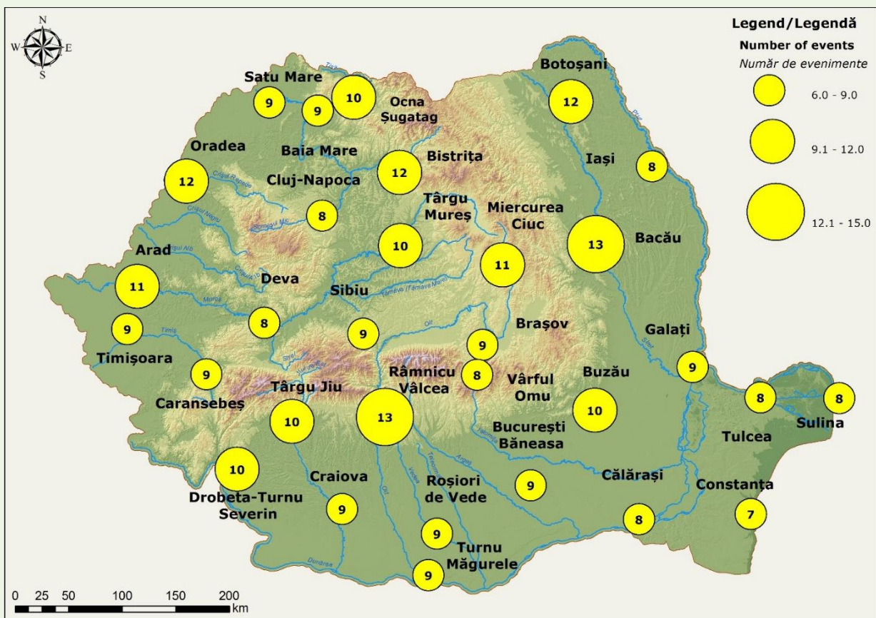
Fig. 1.128. Spatial distribution of maximum annual number of extremely severe heat waves/warm spells Distribuția spațială a numărului maxim anual al valurilor de căldură/periodelor calde extrem de severe
