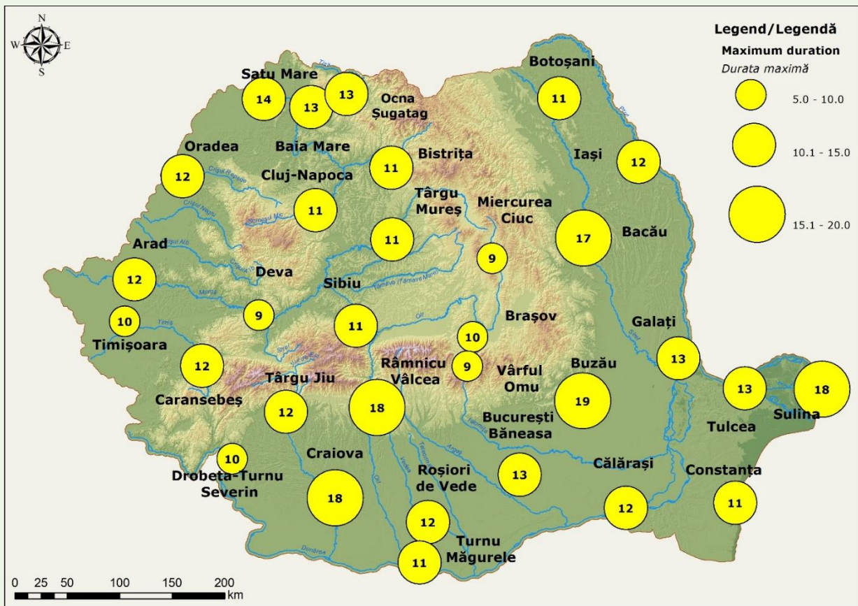
Fig. 1.127. Spatial distribution of maximum annual duration of extremely severe heat waves/warm spells Distribuția spațială a duratei maxime anuale a valurilor de căldură/periodelor calde extrem de severe
