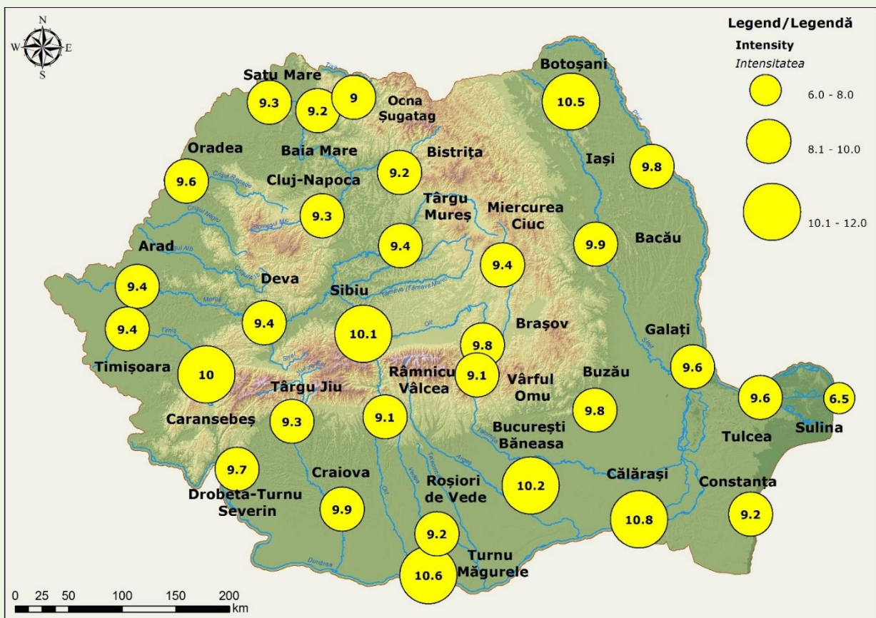
Fig. 1.130. Spatial distribution of mean annual intensity of extremely severe heat waves/warm spells Distribuția spațială a intensității medii anuale a valurilor de căldură/perioadelor calde extrem de severe
