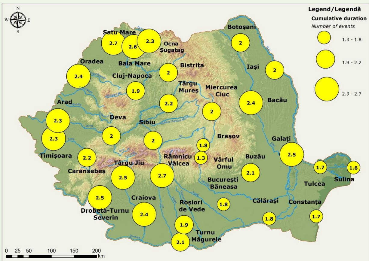
Fig. 1.132. Spatial distribution of mean annual number of extremely severe heat waves/warm spells Distribuția spațială a numărului mediu anual al valurilor de căldură/perioadelor calde extrem de severe
