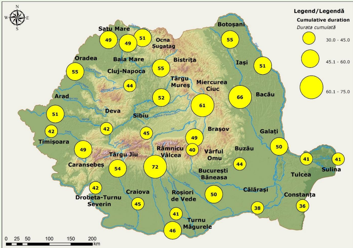
Fig. 1.125. Spatial distribution of maximum annual cumulative duration of extremely severe heat waves/warm spells Distribuția spațială a duratei cumulate maxime anuale a valurilor de căldură/periodelor calde extrem de severe
