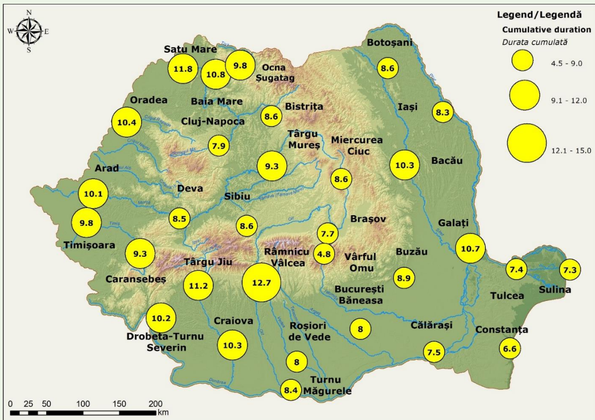
Fig. 1.129. Spatial distribution of mean annual cumulative duration of extremely severe heat waves/warm spells Distribuția spațială a duratei cumulate medii anuale a valurilor de căldură/perioadelor calde extrem de severe
